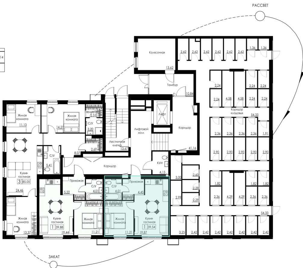
Секция 13 | 1 этаж
